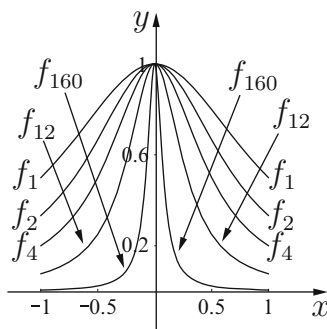
Fig. 9.7. f_n(x) = 1/(1+nx^2) on (-1, 1) .
