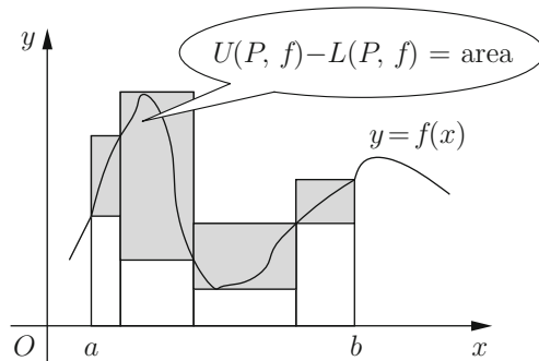
Fig. 6.7. U(P, f) - L(P, f) = \text{area} \geq 0 .
